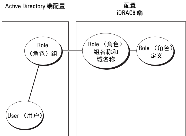
图 6-3. 用 Microsoft Active Directory 和标准架构配置 iDRAC6
